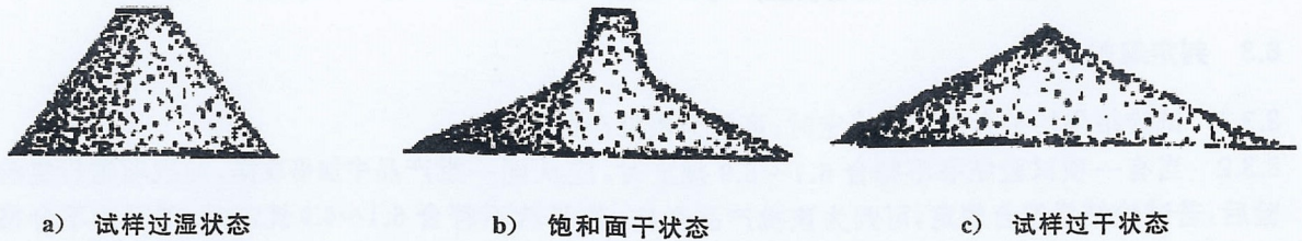
图5 机制砂饱和面干状态示意图
